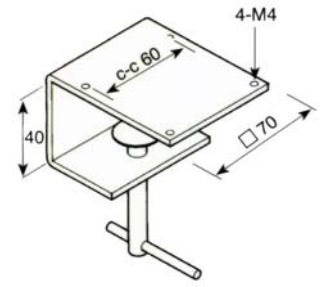
300-CD Table Edge Clamp
